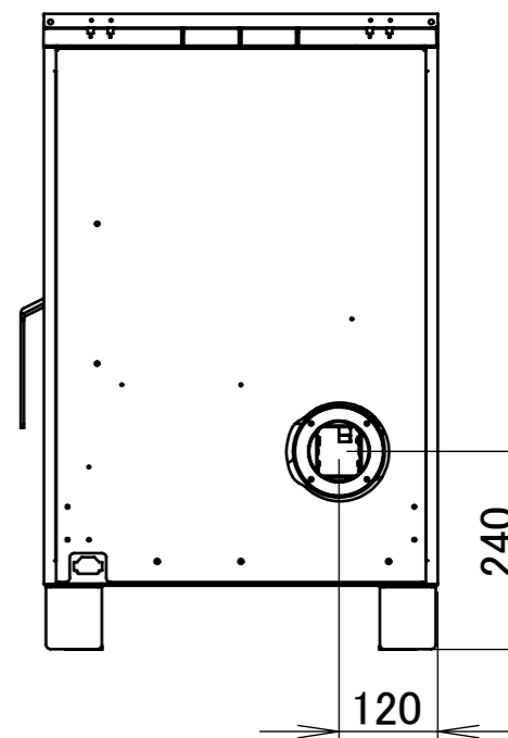
SAIKAI SS-5 Plus 外観寸法図
