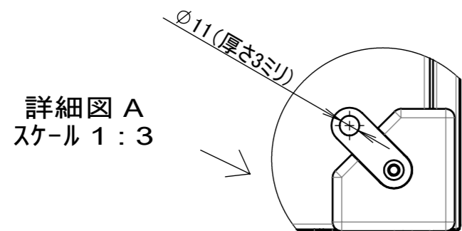
【アンカー穴寸法】
