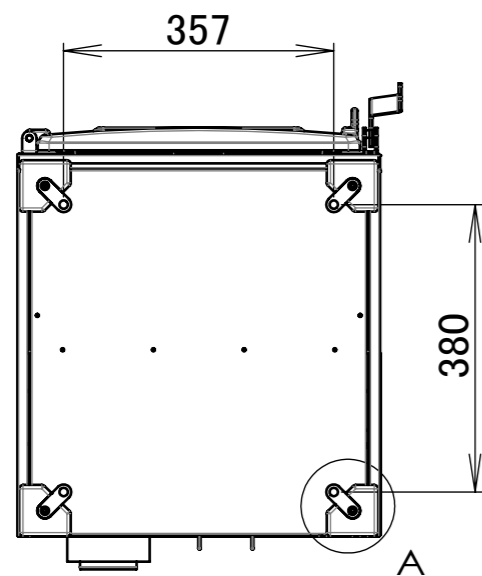
【アンカー穴寸法】
